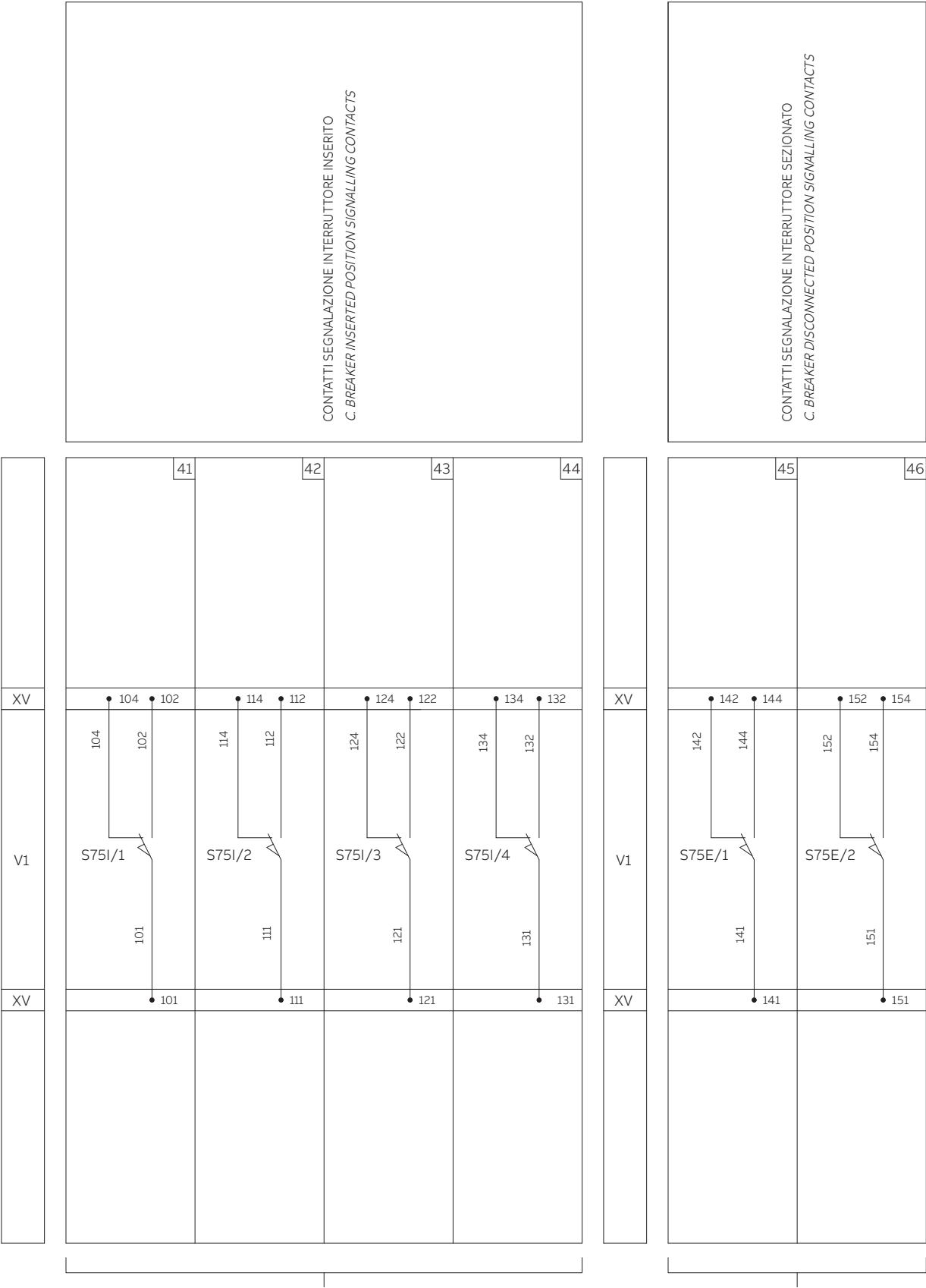
SOLO PER INTERRUTTORI IN ESECUZIONE RIMOVIBILE O ESTRAIBILE ONLY FOR PLUG-IN OR WITHDRAWABLE VERSION C.BREAKER
