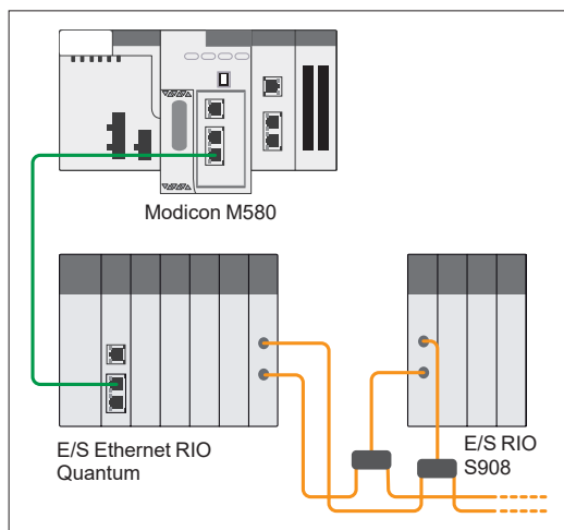
Exemple d'architecture autonome
