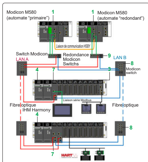
Architecture redondante à haute disponibilité
