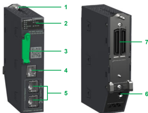
BMENOR2200H, faces avant et arrière
