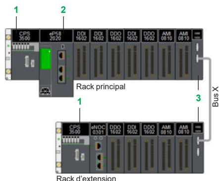
Architecture avec E/S locales : équipements sur E/S locales
