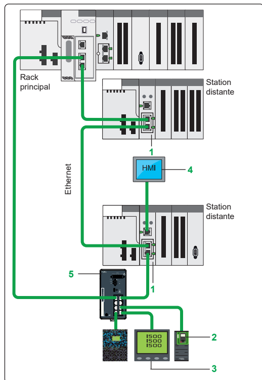
Architecture avec E/S distantes : équipements sur E/S distantes
