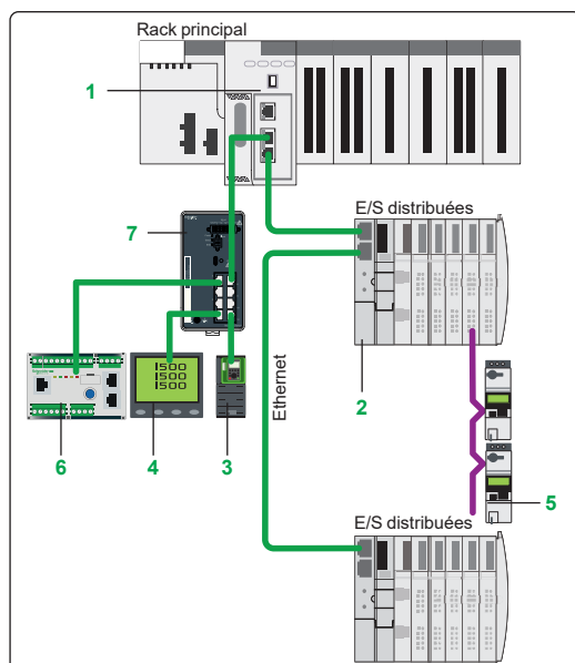
Architecture avec entrées/sorties distribuées : équipements distribués sur Ethernet avec switch Modicon
