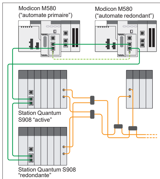
Exemple d'architecture à haute disponibilité
