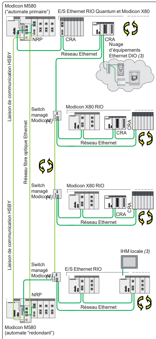
Architecture redondante d'entrées/sorties Ethernet Modicon M580, longue distance
