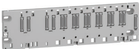
Fond de panier pour alimentation redondante, 6 emplacements
