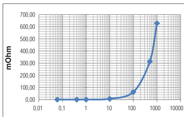
Impédance d'insertion
