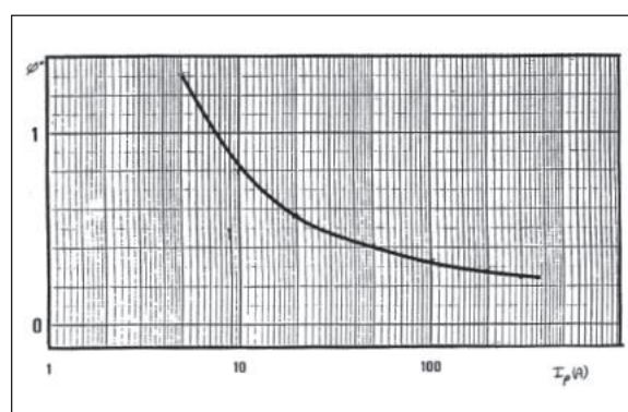
Déphasage
