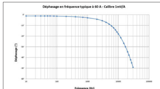
Déphasage fréquentiel
